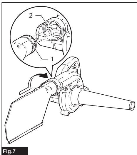
► 1. Entrée de sac à poussières 2. Sortie de souffleur
